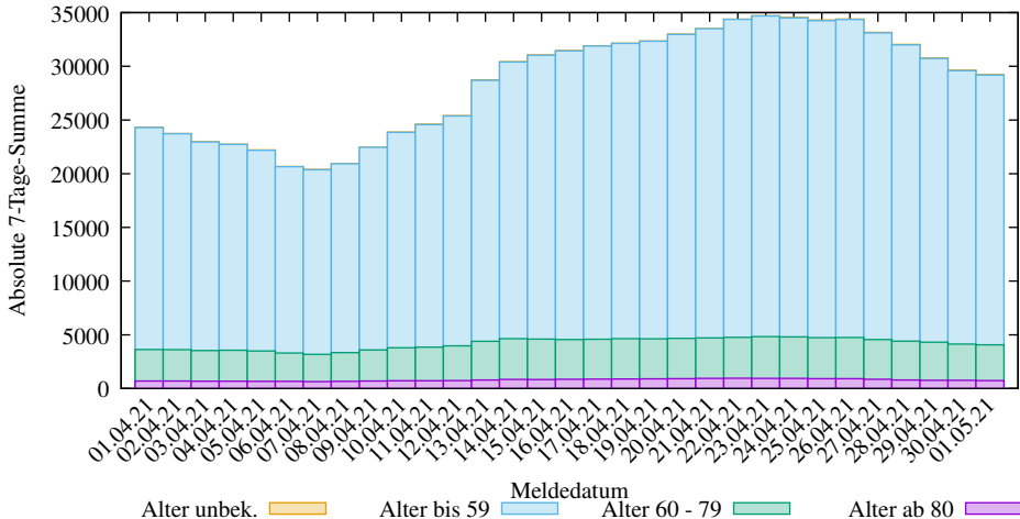
Abs. 7-Tage-Summen der neuen COVID-19 Infizierten in Nordrhein-Westf. (2025-03-09/2104, D. Lippold, https://covid19-de-stats.sourceforge.io/ Lizenz: CC BY-ND 4.0, Daten: Robert Koch-Institut (RKI), dl-de/by-2-0)
