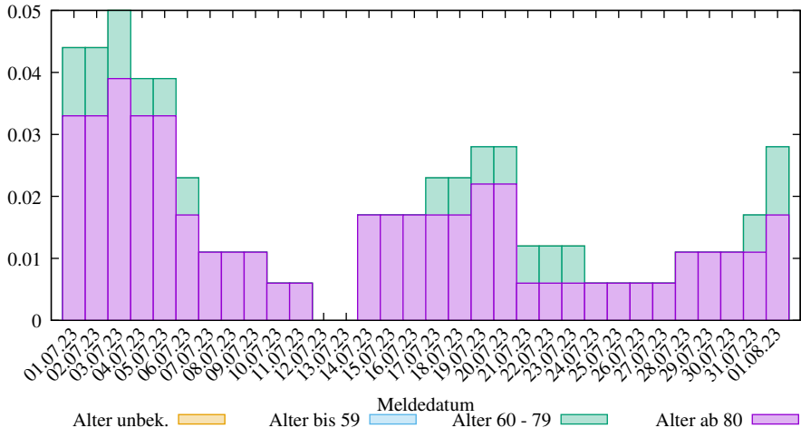
Rel. 7-Tage-Summe der neuen COVID-19 Verstorbenen in Nordrhein-Westf. (2025-03-09/2307, D. Lippold, https://covid19-de-stats.sourceforge.io/ Lizenz: CC BY-ND 4.0, Daten: Robert Koch-Institut (RKI), dl-de/by-2-0)
