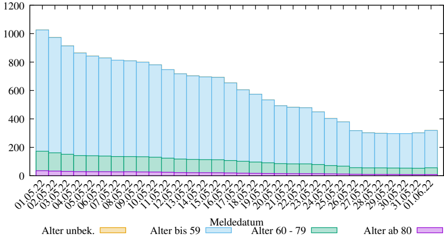
Rel. 7-Tage-Summe der neuen COVID-19 Infizierten in Niedersachsen (2025-03-09/2205, D. Lippold, https://covid19-de-stats.sourceforge.io/ Lizenz: CC BY-ND 4.0, Daten: Robert Koch-Institut (RKI), dl-de/by-2-0)
