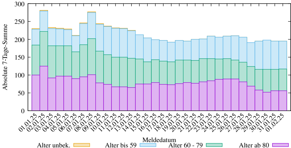
Abs. 7-Tage-Summen der neuen COVID-19 Infizierten in Niedersachsen (2025-03-09/2501, D. Lippold, https://covid19-de-stats.sourceforge.io/ Lizenz: CC BY-ND 4.0, Daten: Robert Koch-Institut (RKI), dl-de/by-2-0)
