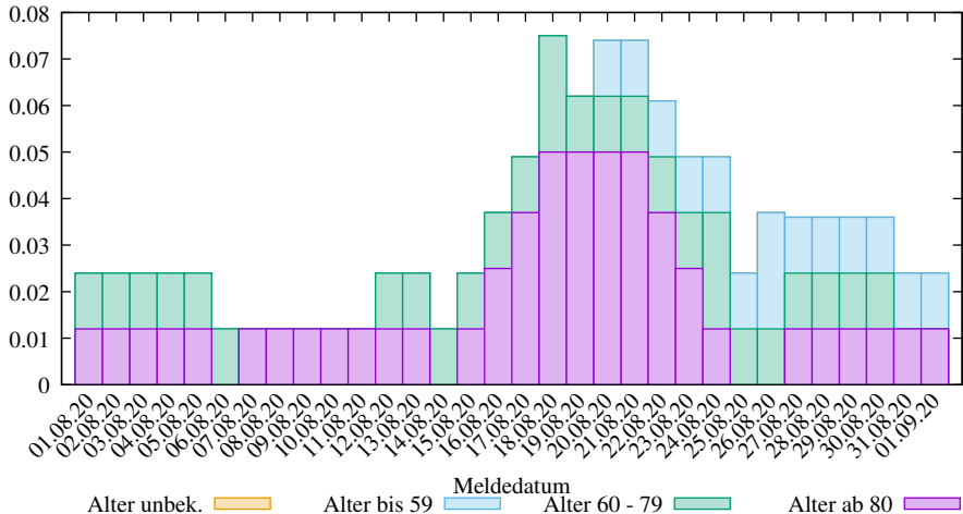
Rel. 7-Tage-Summe der neuen COVID-19 Verstorbenen in Niedersachsen (2025-03-09/2008, D. Lippold, https://covid19-de-stats.sourceforge.io/ Lizenz: CC BY-ND 4.0, Daten: Robert Koch-Institut (RKI), dl-de/by-2-0)
