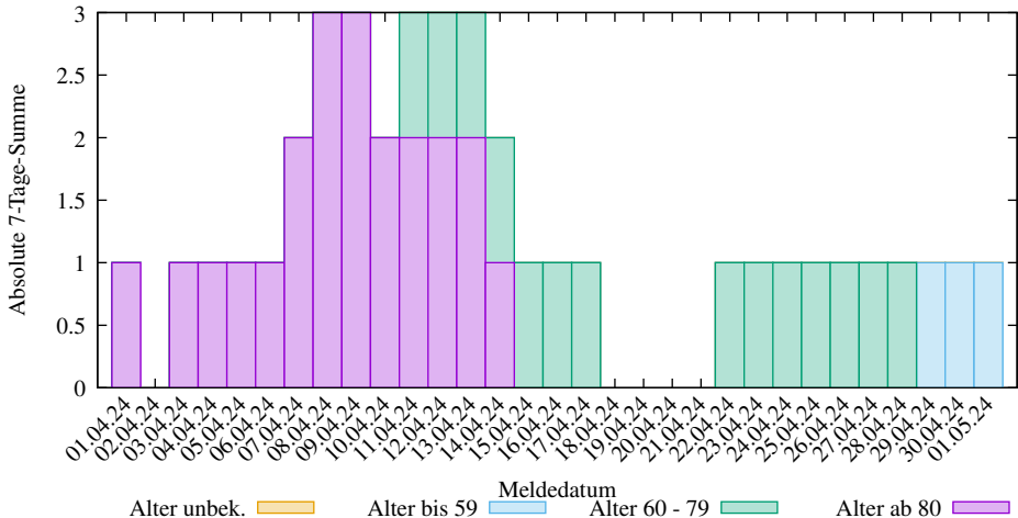
Abs. 7-Tage-Summen der neuen COVID-19 Verstorbenen in Niedersachsen (2025-03-09/2404, D. Lippold, https://covid19-de-stats.sourceforge.io/ Lizenz: CC BY-ND 4.0, Daten: Robert Koch-Institut (RKI), dl-de/by-2-0)
