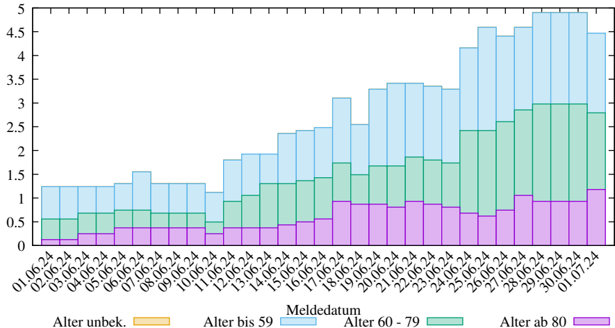
Rel. 7-Tage-Summe der neuen COVID-19 Infizierten in Meckl.-Vorpom. (2025-03-09/2406, D. Lippold, https://covid19-de-stats.sourceforge.io/ Lizenz: CC BY-ND 4.0, Daten: Robert Koch-Institut (RKI), dl-de/by-2-0)
