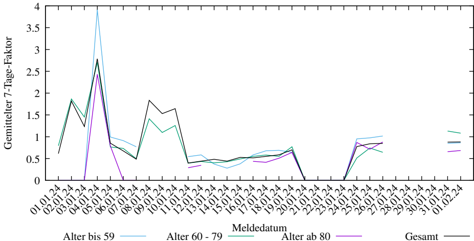
7-Tage-Faktoren der neuen COVID-19 Infizierten in Meckl.-Vorpom. (2025-03-09/2401, D. Lippold, https://covid19-de-stats.sourceforge.io/ Lizenz: CC BY-ND 4.0, Daten: Robert Koch-Institut (RKI), dl-de/by-2-0)
