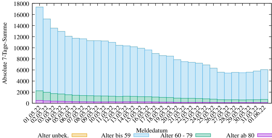
Abs. 7-Tage-Summen der neuen COVID-19 Infizierten in Hamburg (2025-03-09/2205, D. Lippold, https://covid19-de-stats.sourceforge.io/ Lizenz: CC BY-ND 4.0, Daten: Robert Koch-Institut (RKI), dl-de/by-2-0)
