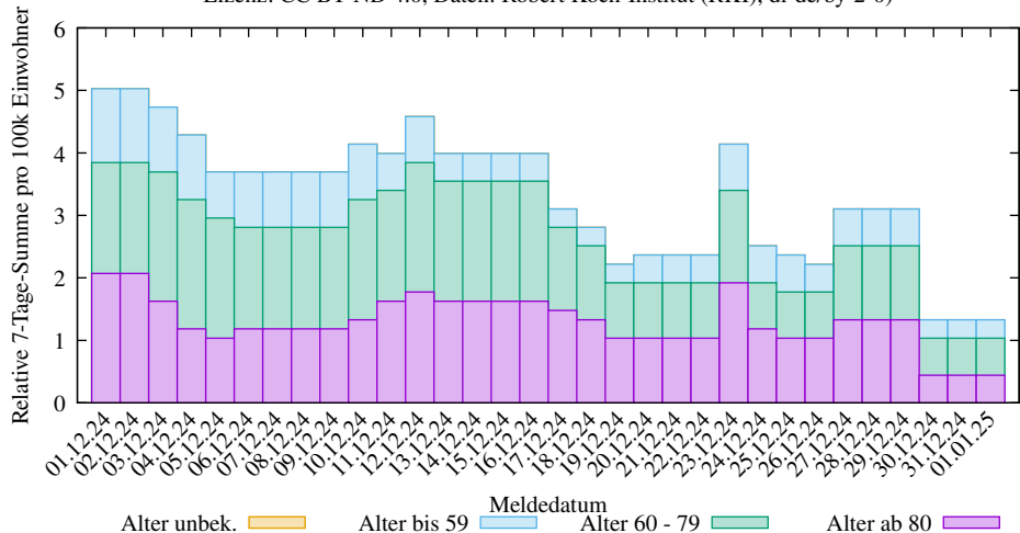
Rel. 7-Tage-Summe der neuen COVID-19 Infizierten in Bremen (2025-03-09/2412, D. Lippold, https://covid19-de-stats.sourceforge.io/ Lizenz: CC BY-ND 4.0, Daten: Robert Koch-Institut (RKI), dl-de/by-2-0)
