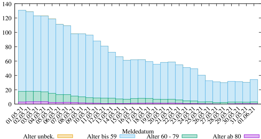
Rel. 7-Tage-Summe der neuen COVID-19 Infizierten in Bremen (2025-03-09/2105, D. Lippold, https://covid19-de-stats.sourceforge.io/ Lizenz: CC BY-ND 4.0, Daten: Robert Koch-Institut (RKI), dl-de/by-2-0)
