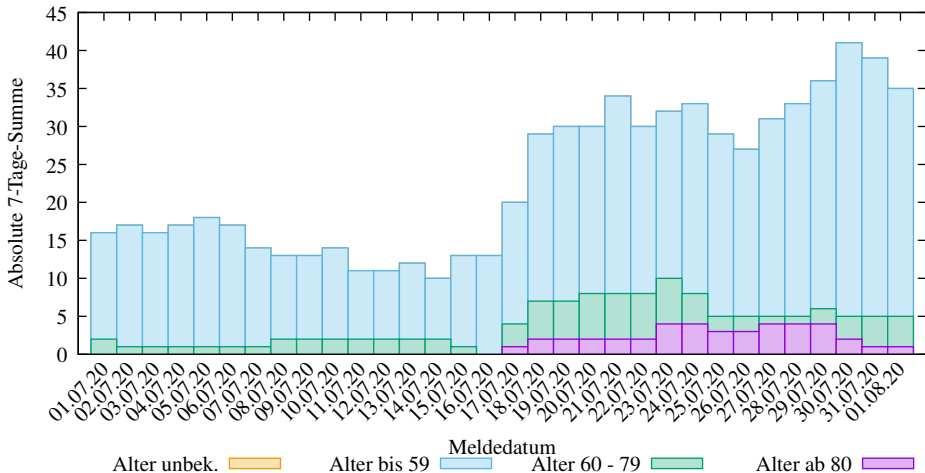
Abs. 7-Tage-Summen der neuen COVID-19 Infizierten in Bremen (2025-03-09/2007, D. Lippold, https://covid19-de-stats.sourceforge.io/ Lizenz: CC BY-ND 4.0, Daten: Robert Koch-Institut (RKI), dl-de/by-2-0)
