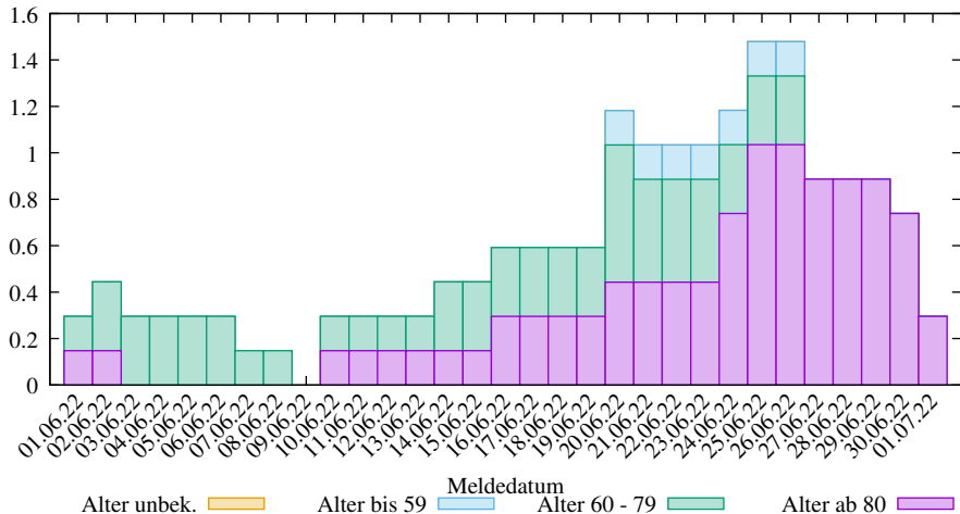
Rel. 7-Tage-Summe der neuen COVID-19 Verstorbenen in Bremen (2025-03-09/2206, D. Lippold, https://covid19-de-stats.sourceforge.io/ ) Lizenz: CC BY-ND 4.0, Daten: Robert Koch-Institut (RKI), dl-de/by-2-0)
