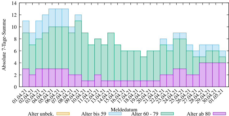
Abs. 7-Tage-Summen der neuen COVID-19 Verstorbenen in Bremen (2025-03-09/2104, D. Lippold, https://covid19-de-stats.sourceforge.io/ Lizenz: CC BY-ND 4.0, Daten: Robert Koch-Institut (RKI), dl-de/by-2-0)
