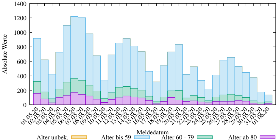
Einzelwerte der neuen COVID-19 Infizierten in Deutschland gesamt (2025-03-09/2005, D. Lippold, https://covid19-de-stats.sourceforge.io/ Lizenz: CC BY-ND 4.0, Daten: Robert Koch-Institut (RKI), dl-de/by-2-0)
