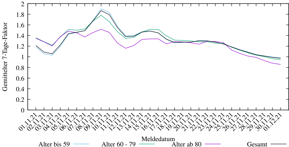
7-Tage-Faktoren der neuen COVID-19 Infizierten in Deutschland gesamt (2025-03-09/2111, D. Lippold, https://covid19-de-stats.sourceforge.io/ Lizenz: CC BY-ND 4.0, Daten: Robert Koch-Institut (RKI), dl-de/by-2-0)
