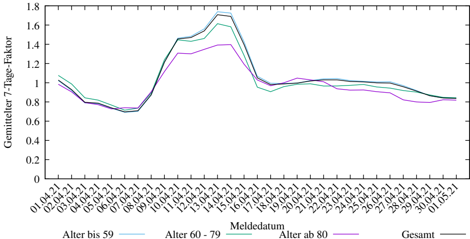
7-Tage-Faktoren der neuen COVID-19 Infizierten in Deutschland gesamt (2025-03-09/2104, D. Lippold, https://covid19-de-stats.sourceforge.io/ Lizenz: CC BY-ND 4.0, Daten: Robert Koch-Institut (RKI), dl-de/by-2-0)
