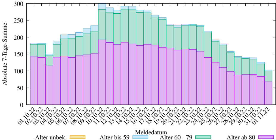
Abs. 7-Tage-Summen der neuen COVID-19 Verstorbenen in Bayern (2025-03-09/2210, D. Lippold, https://covid19-de-stats.sourceforge.io/ Lizenz: CC BY-ND 4.0, Daten: Robert Koch-Institut (RKI), dl-de/by-2-0)
