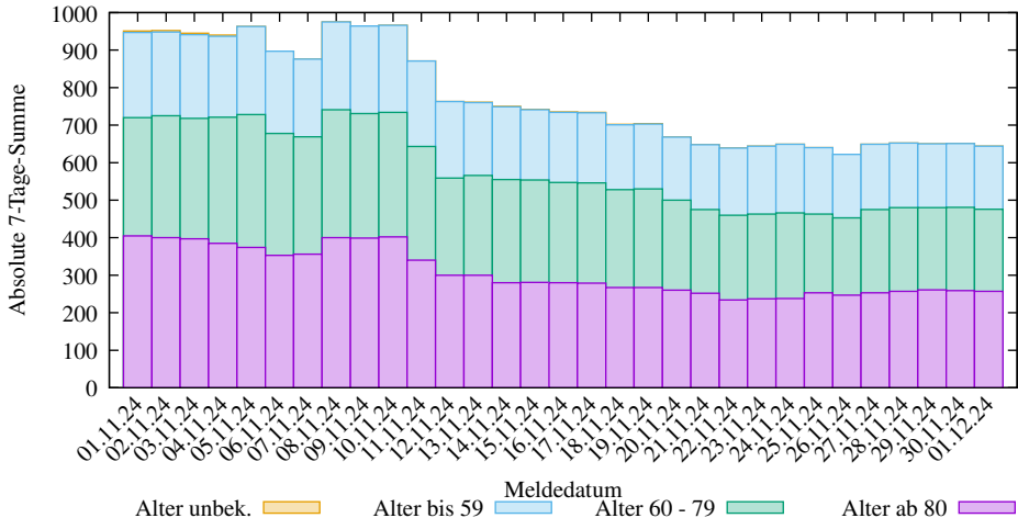
Abs. 7-Tage-Summen der neuen COVID-19 Infizierten in Baden-Württemberg (2025-03-09/2411, D. Lippold, https://covid19-de-stats.sourceforge.io/ Lizenz: CC BY-ND 4.0, Daten: Robert Koch-Institut (RKI), dl-de/by-2-0)
