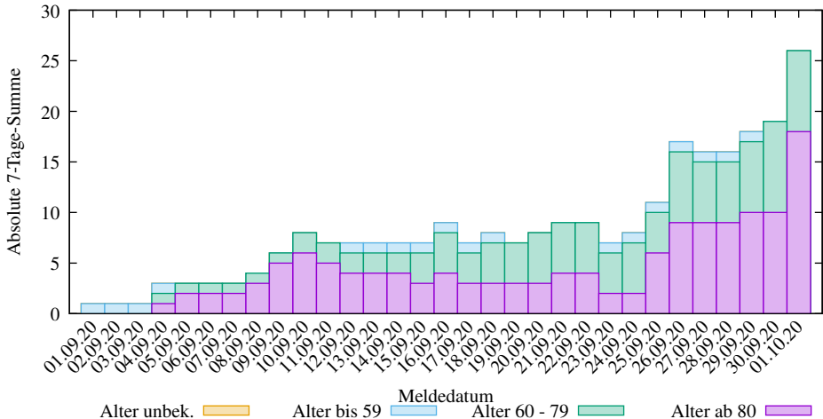
Abs. 7-Tage-Summen der neuen COVID-19 Verstorbenen in Baden-Württemberg (2025-03-09/2009, D. Lippold, https://covid19-de-stats.sourceforge.io/ Lizenz: CC BY-ND 4.0, Daten: Robert Koch-Institut (RKI), dl-de/by-2-0)
