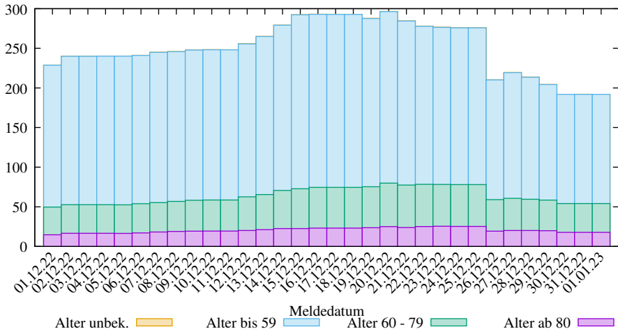
Rel. 7-Tage-Summe der neuen COVID-19 Infizierten in Berlin (2025-03-09/2212, D. Lippold, https://covid19-de-stats.sourceforge.io/ Lizenz: CC BY-ND 4.0, Daten: Robert Koch-Institut (RKI), dl-de/by-2-0)
