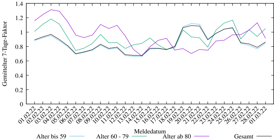
7-Tage-Faktoren der neuen COVID-19 Infizierten in Berlin (2025-03-09/2202, D. Lippold, https://covid19-de-stats.sourceforge.io/ Lizenz: CC BY-ND 4.0, Daten: Robert Koch-Institut (RKI), dl-de/by-2-0)
