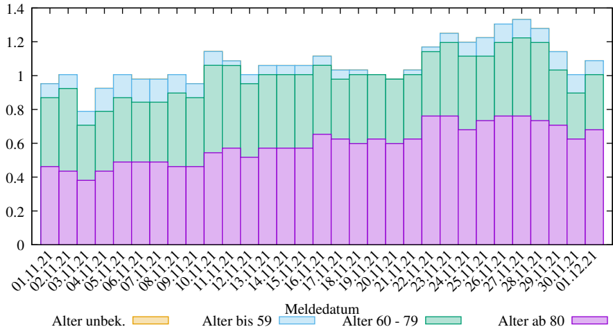
Rel. 7-Tage-Summe der neuen COVID-19 Verstorbenen in Berlin (2025-03-09/2111, D. Lippold, https://covid19-de-stats.sourceforge.io/ Lizenz: CC BY-ND 4.0, Daten: Robert Koch-Institut (RKI), dl-de/by-2-0)
