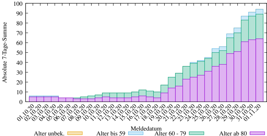
Abs. 7-Tage-Summen der neuen COVID-19 Verstorbenen in Berlin (2025-03-09/2010, D. Lippold, https://covid19-de-stats.sourceforge.io/ Lizenz: CC BY-ND 4.0, Daten: Robert Koch-Institut (RKI), dl-de/by-2-0)
