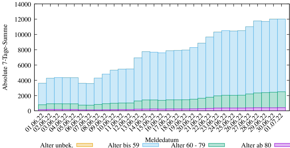
Abs. 7-Tage-Summen der neuen COVID-19 Infizierten in Brandenburg (2025-03-09/2206, D. Lippold, https://covid19-de-stats.sourceforge.io/ Lizenz: CC BY-ND 4.0, Daten: Robert Koch-Institut (RKI), dl-de/by-2-0)
