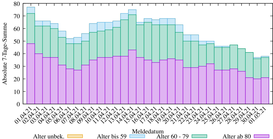
Abs. 7-Tage-Summen der neuen COVID-19 Verstorbenen in Brandenburg (2025-03-09/2104, D. Lippold, https://covid19-de-stats.sourceforge.io/ Lizenz: CC BY-ND 4.0, Daten: Robert Koch-Institut (RKI), dl-de/by-2-0)
