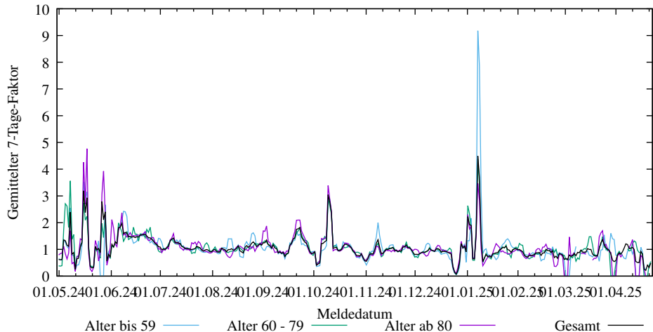
7-Tage-Faktoren der neuen COVID-19 Infizierten in Deutschland gesamt (2025-04-26/Short, D. Lippold, https://covid19-de-stats.sourceforge.io/ Lizenz: CC BY-ND 4.0, Daten: Robert Koch-Institut (RKI), dl-de/by-2-0)
