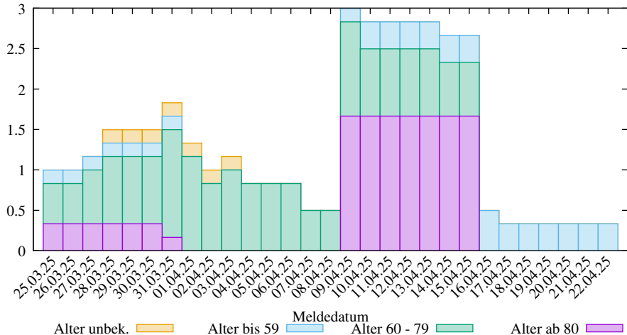
Rel. 7-Tage-Summe der neuen COVID-19 Infizierten in LK Rhein-Sieg-Kreis (2025-04-26/Limit, D. Lippold, https://covid19-de-stats.sourceforge.io/ Lizenz: CC BY-ND 4.0, Daten: Robert Koch-Institut (RKI), dl-de/by-2-0)
