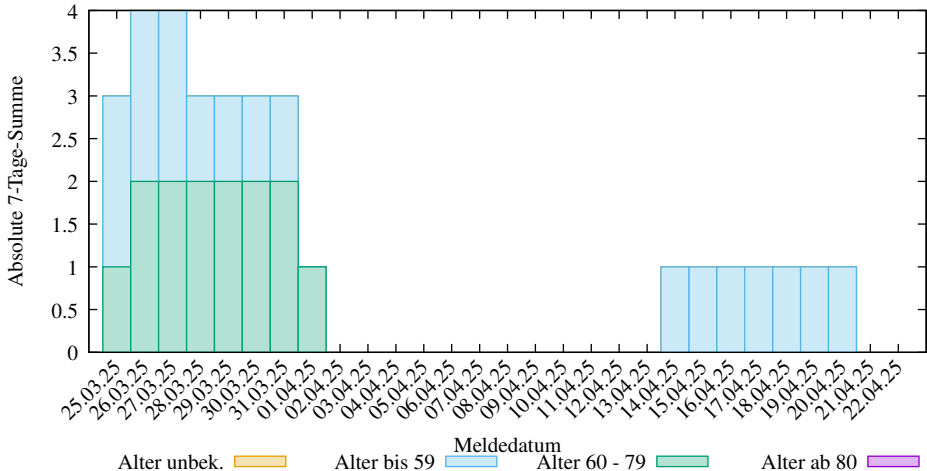
Abs. 7-Tage-Summen der neuen COVID-19 Infizierten in LK Steinburg (2025-04-26/Limit, D. Lippold, https://covid19-de-stats.sourceforge.io/ ) Lizenz: CC BY-ND 4.0, Daten: Robert Koch-Institut (RKI), dl-de/by-2-0)
